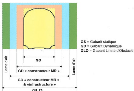
Description du Gabarit limite d'obstacle (GLO)
